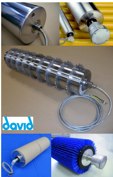
Trummotorer TM60 .....TM 800
